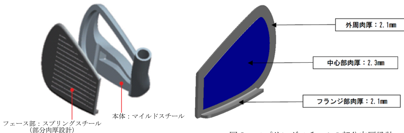
図2：スプリングスチールの部分肉厚設計
