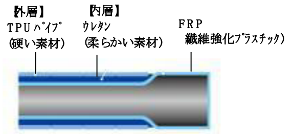
【バット打球部断面構造】
