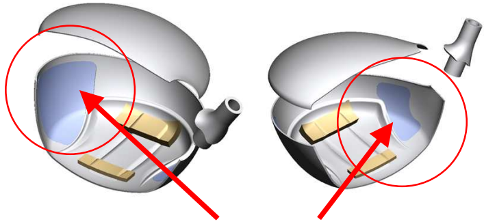
図2：ヘッド内側のトゥ・ヒール部分の軽量化(約7.5g)
