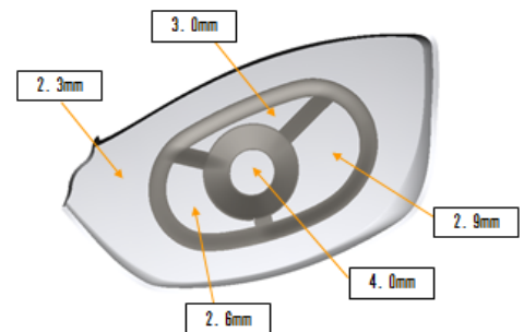
図4：フェース肉厚の5分割イメージ
