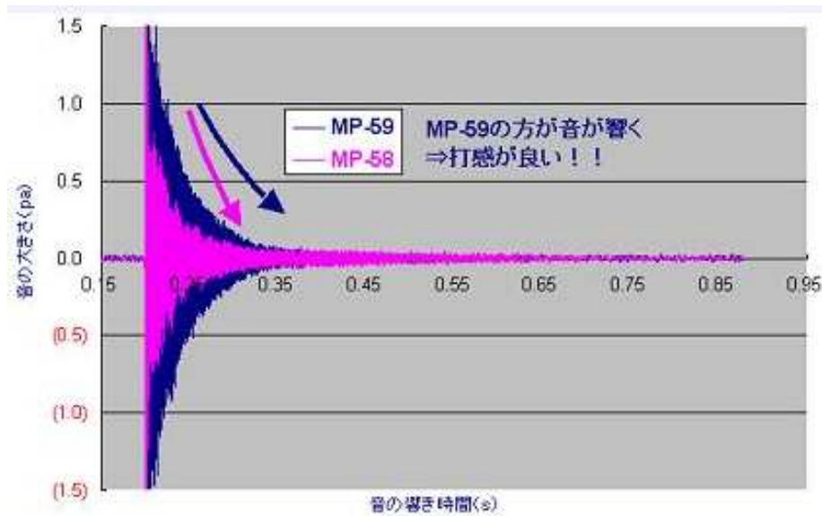
図2：「ミズノMP-59」と「ミズノMP-58」の音の大きさと響く時間のグラフ
