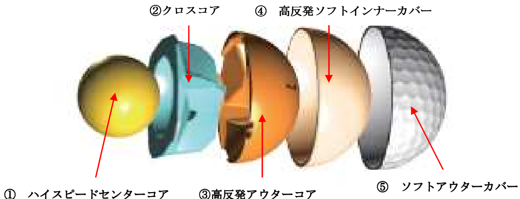
図2：「ミズノ J P X」ゴルフボールの5ピース構造図
