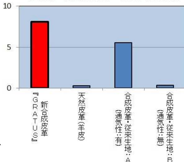
図1：新合成皮革『GRATUS』と天然皮革、 従来の合成皮革の通気度を比較したグラフ
