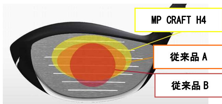
図2：弊社従来品に比べフェース上方向に拡げたスイートエリアの位置（イメージ）
