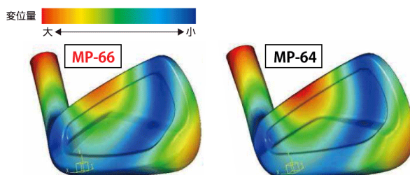
インパクト時のヘッド最大変位画像
