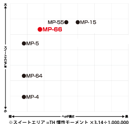
MP アイアンの設計値比較 (No.6)
